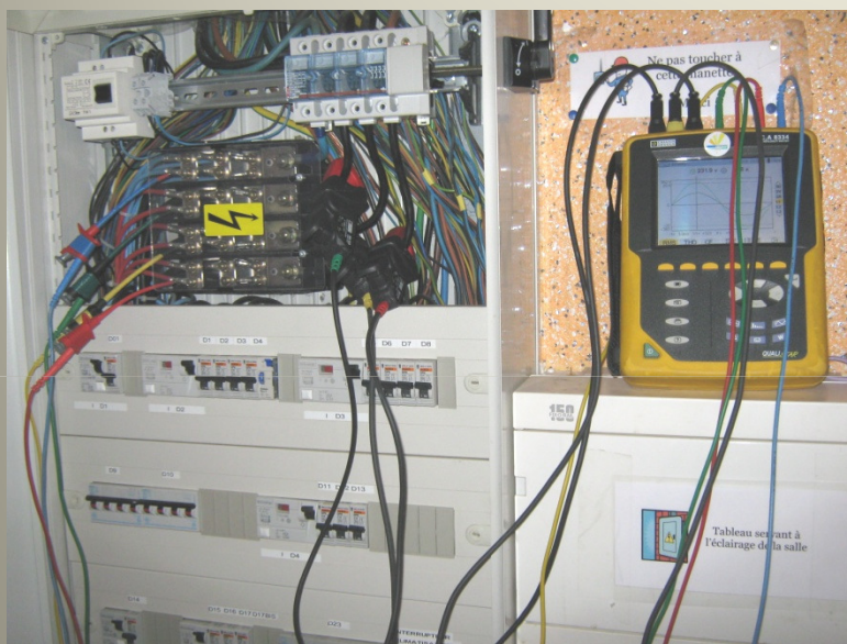
Instrumentation d'une armoire électrique
